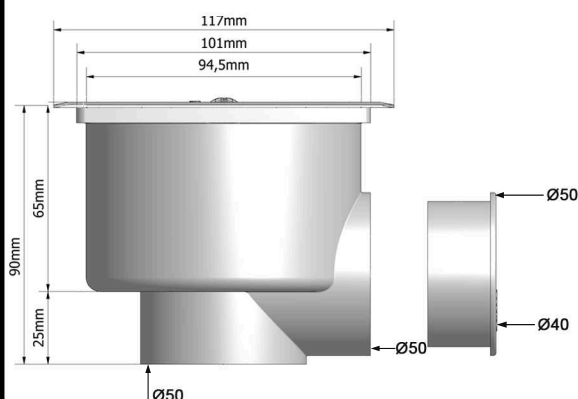
COTAS
